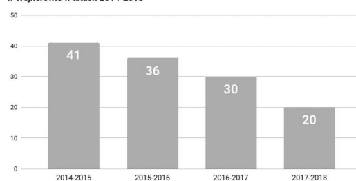
Częstotliwość przekroczeń średniodobowego (24h) stężenia dopuszczalnego pyłu zawieszonego PM 10 (50 µg/m 3 ) w sezonach grzewczych od 1 października do 28 lutego w Wejherowie w latach 2014-2018
