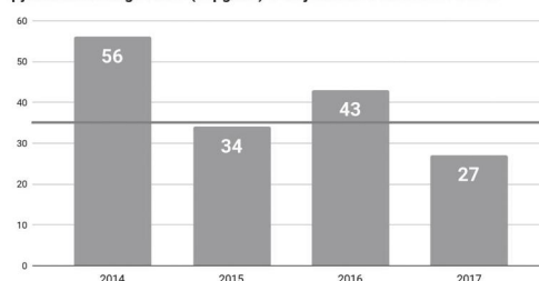
Częstotliwość przekroczeń średniodobowego (24h) stężenia dopuszczalnego pyłu zawieszonego PM10 (50µg/m 3 ) w Wejherowie w latach 2014-2017
